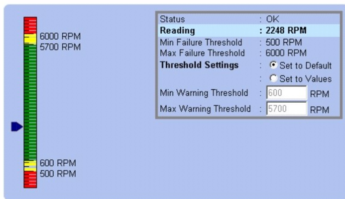
図 5-2 ゲージインジケータ
